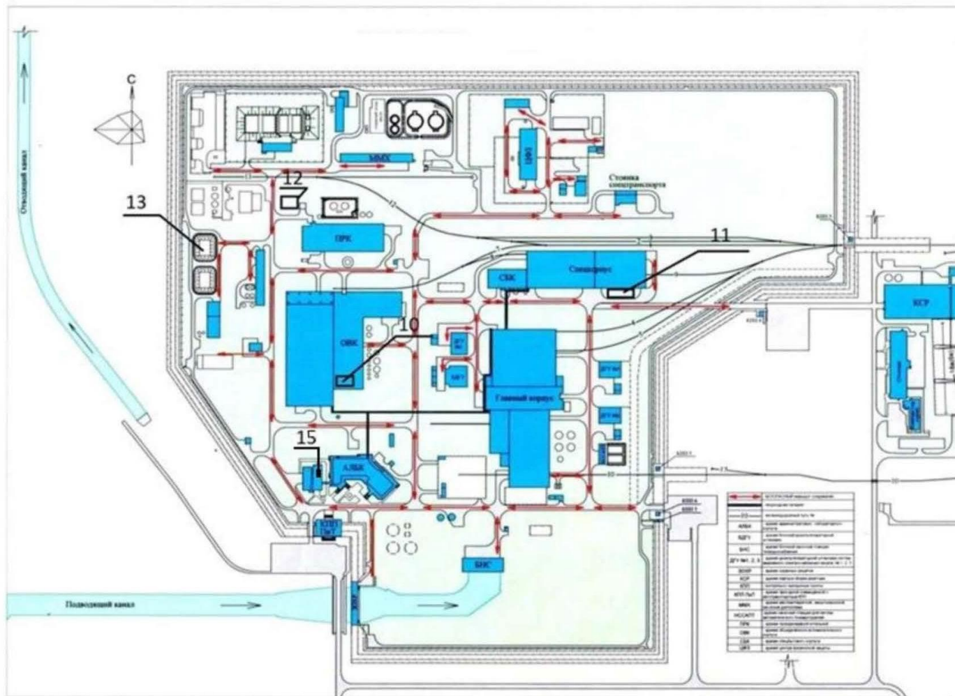
План-схема промплощадки энергоблока № 4 Белоярской АЭС с расположением мест накопления отходов
